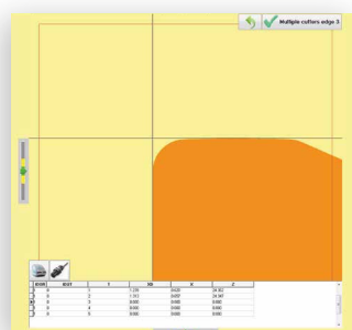
Asse Mobili. Acquisizione automatica delle quote dell'utensile (raggio/altezza). Mobile Axis. Automatic acquisition of tool dimensions (radius/height).
