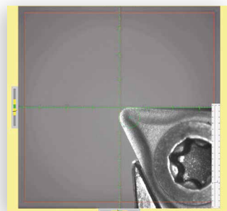
Real View. Ispezione utile per verificare usura e stato del tagliente. Real View. Inspection of tool wear and tool conditions.
