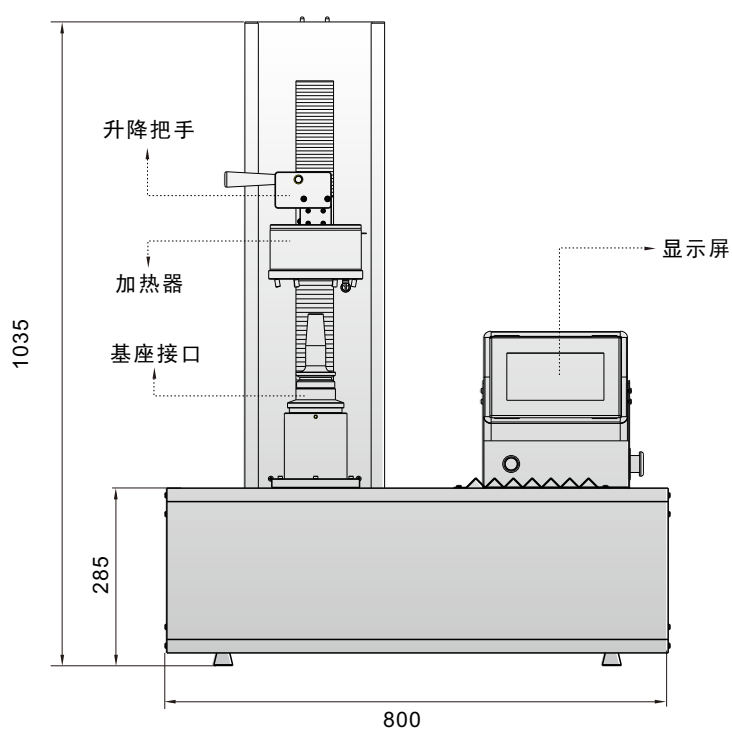
热装机线框图
