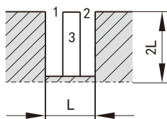
A 深度 > 宽度
