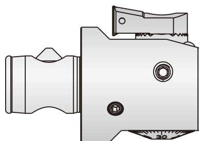
反镗时主轴需反转
