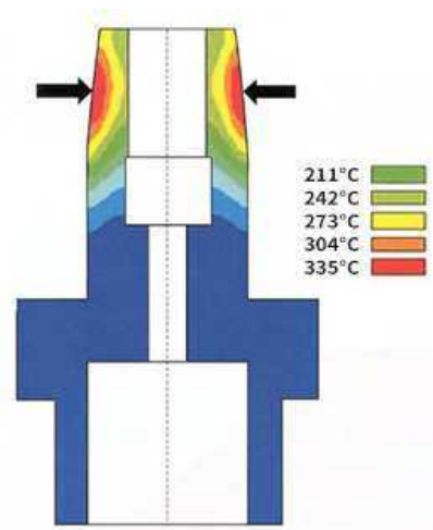
刀柄热成像示意
