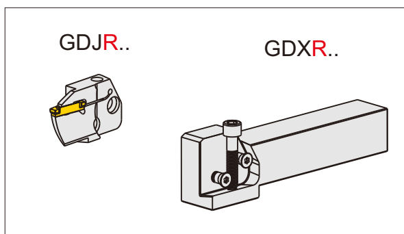
纵向型刀体装配示意
