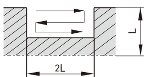
B 宽度 > 深度
